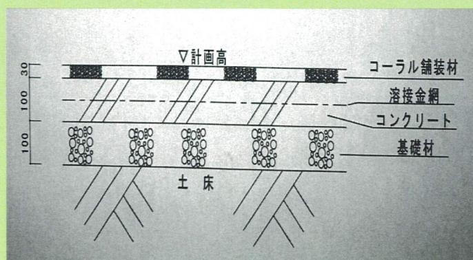
車道仕様断面図
