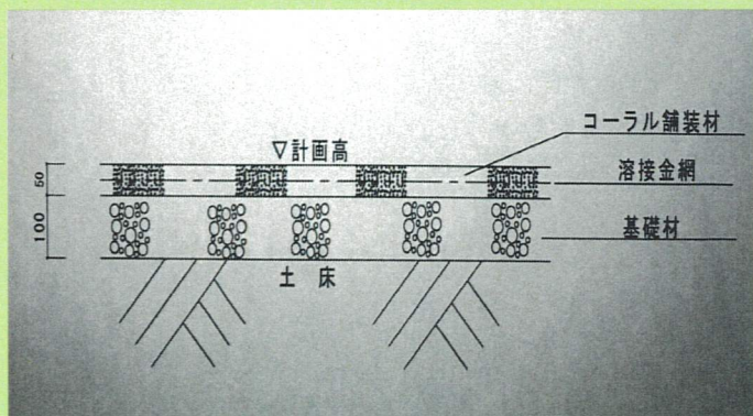
歩道仕様断面図
